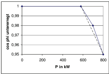
Bild D.1-1: \cos\phi(P) -Kennlinie
