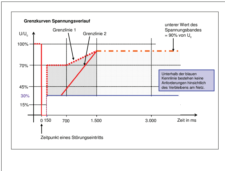
Bild 2.5.1.2-2 Grenzlinien für den Spannungsverlauf am Netzanschlusspunkt für eine Erzeugungsanlage vom Typ 2
