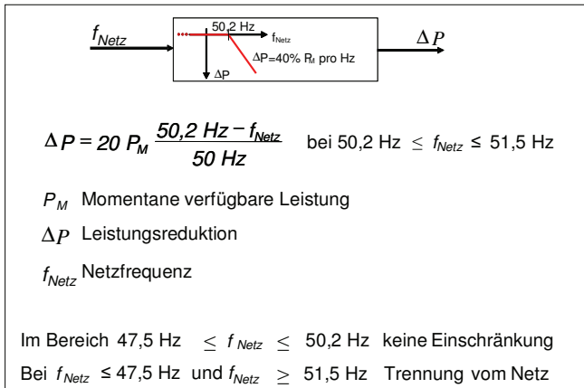
Bild 1 Wirkleistungsreduktion bei Überfrequenz
