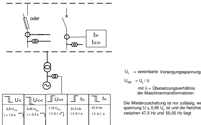
Bild 3.2.3.4-1: Schutzkonzept bei Anschluss von Erzeugungsanlagen im Mittelspannungsnetz
