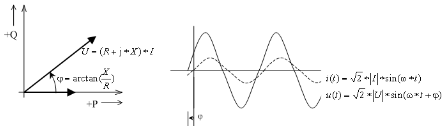
Bild B.4-2: Beispiel: Ohmsch-induktive Last
